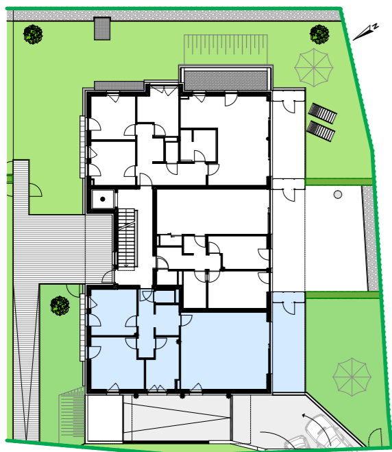
Übersichtsplan, Haus SÜD, EG, Top 1 M 1:400
